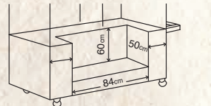
●内部寸法図
